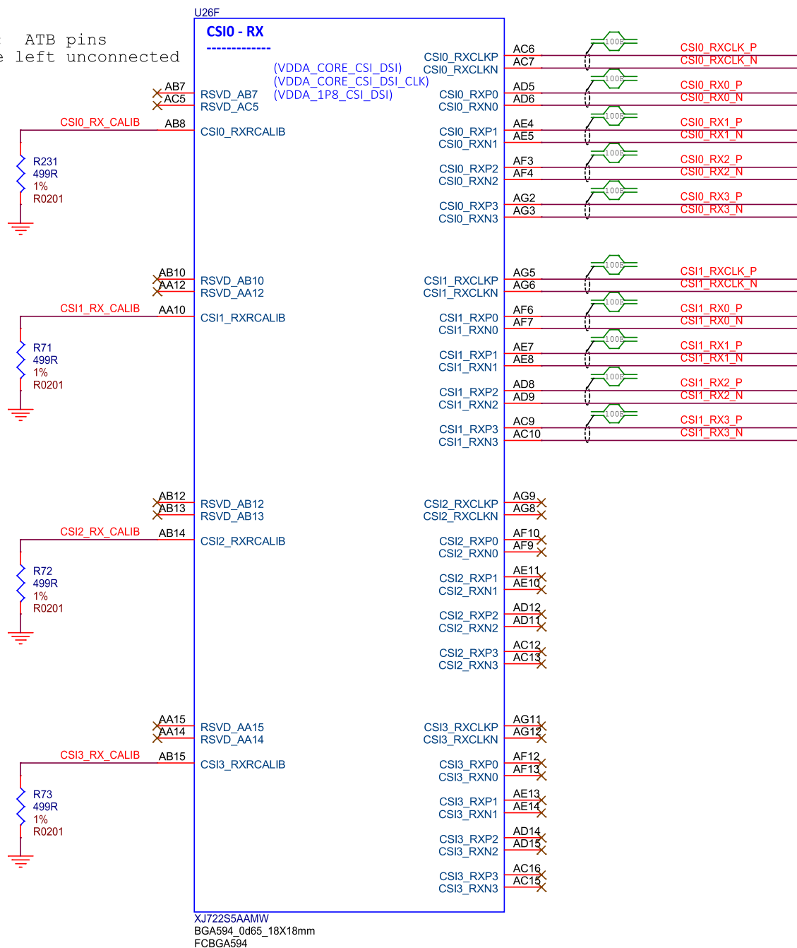
Fig. 3.56: BeagleY-AI SoC CSI1, CSI2, and CSI3
