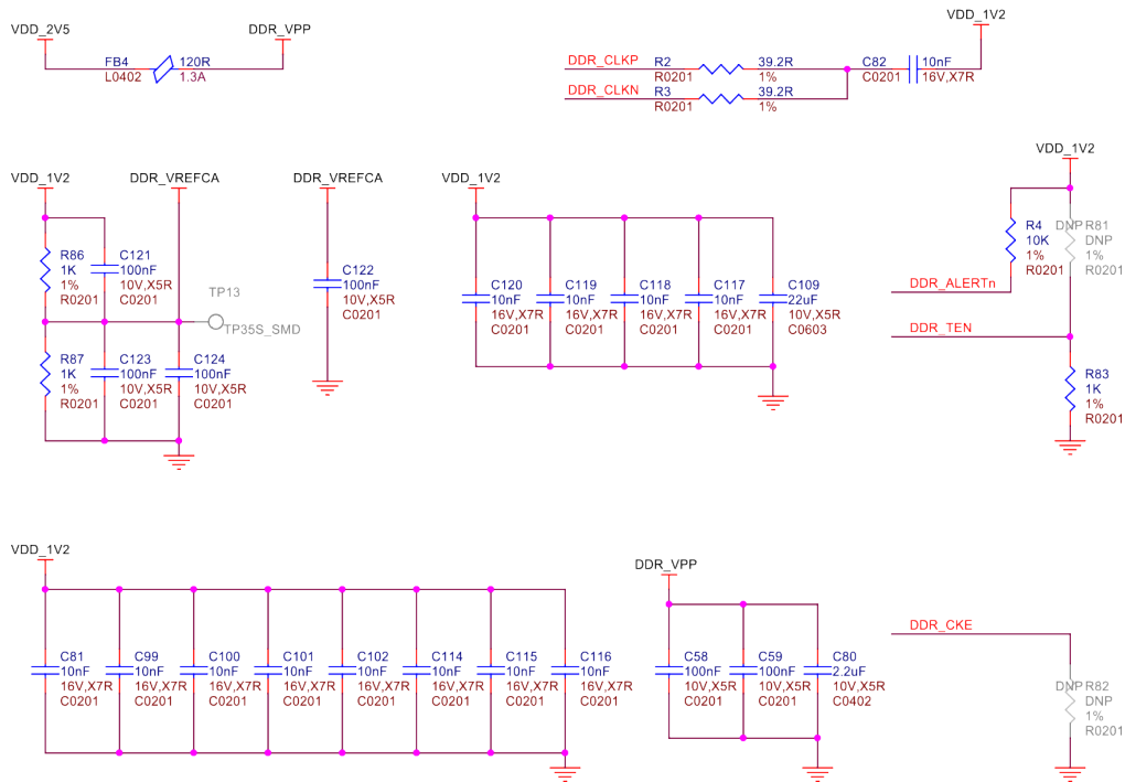
Fig. 3.40: DDR power
